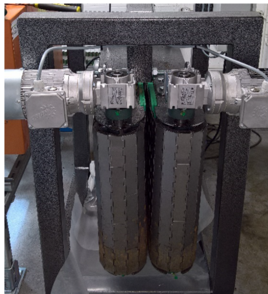
Fig. 3. Hugger crusher (Kuopanportti et al. 2020).
